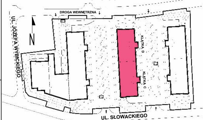
PLAN SYTUACYJNY
