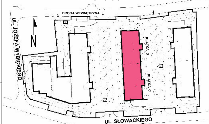
PLAN SYTUACYJNY
